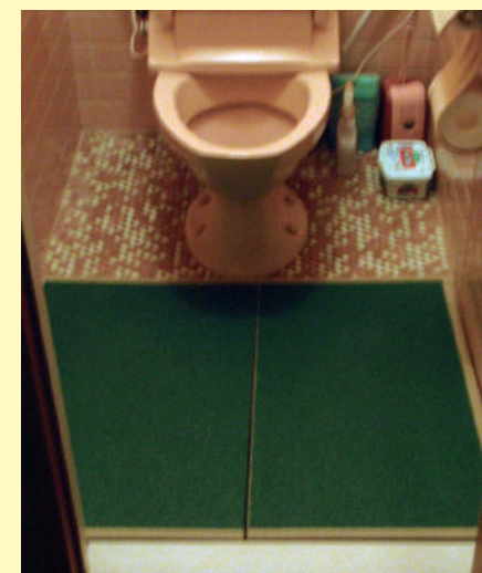
施工後 段差解消スロープ
